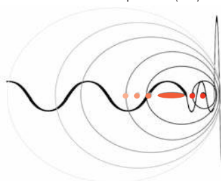
Émetteur en mouvement à la même vitesse que le son (mur)
