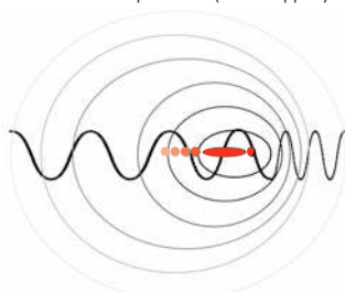
Émetteur en mouvement moins vite que le son (effet Doppler)
